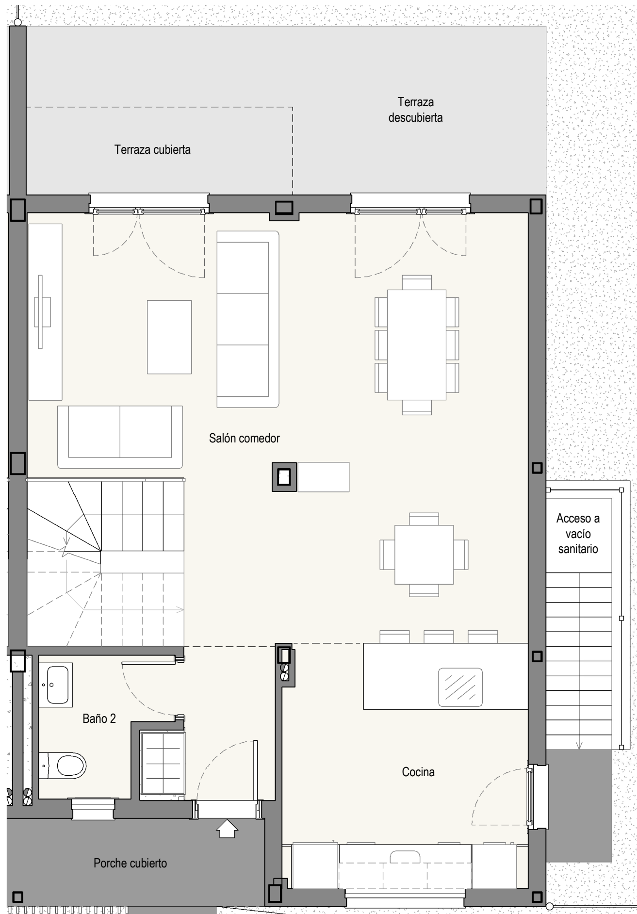
Planta Baja
